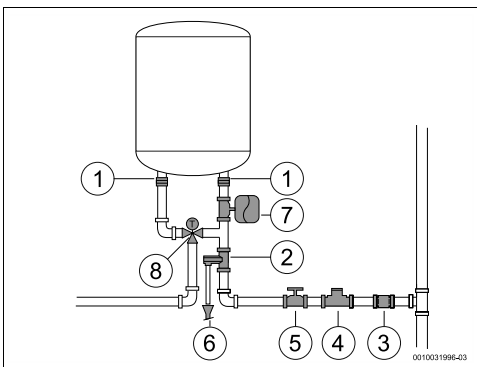
11. ábra Vízbekötés
