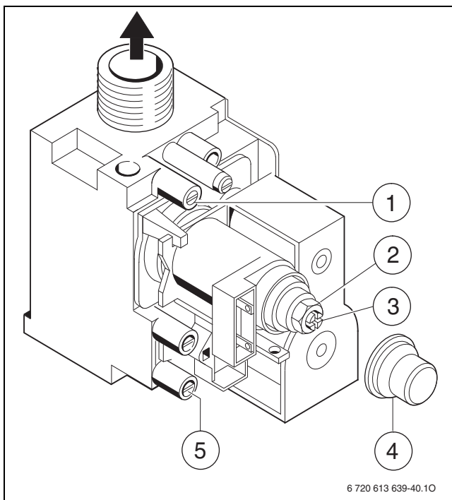
36. ábra Gázarmatúra
