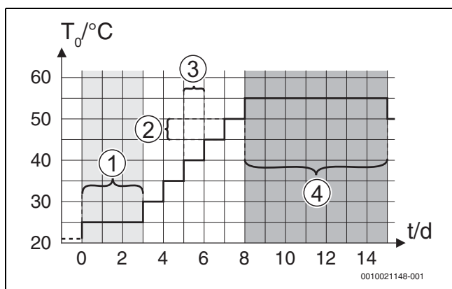
6. ábra Esztrich-szárítási folyamat az alapbeállításokkal a felfűtési fázisban
