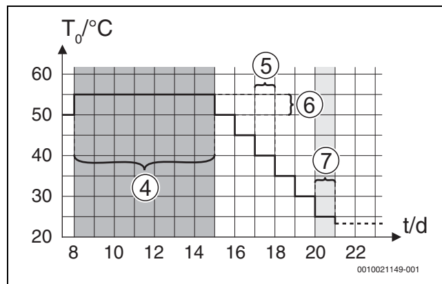
7. ábra Esztrich-szárítási folyamat az alapbeállításokkal a hűtési fázisban
