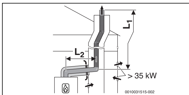
20. ábra B 33 szerinti flexibilis füstgázvezetés kürtőben, környezeti levegőtől függő levegőellátással a koncentrikus levegő- és füstgázvezetésen keresztül a telepítési helyiségben
