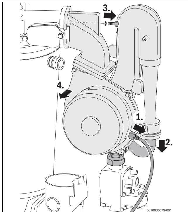
57. ábra A ventilátor és a keverőberendezés kiserelése
