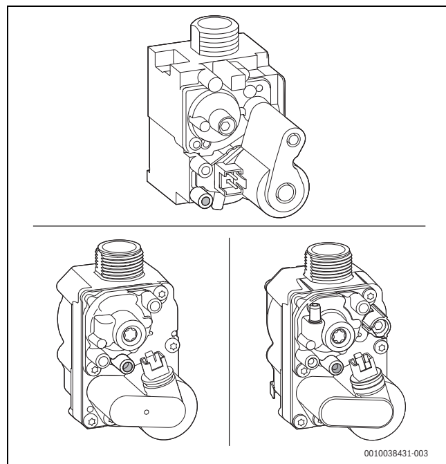
47. ábra Balra fent és lent: nem beállítható gázszerelvény, jobbra lent: beállítható gázszerelvény
