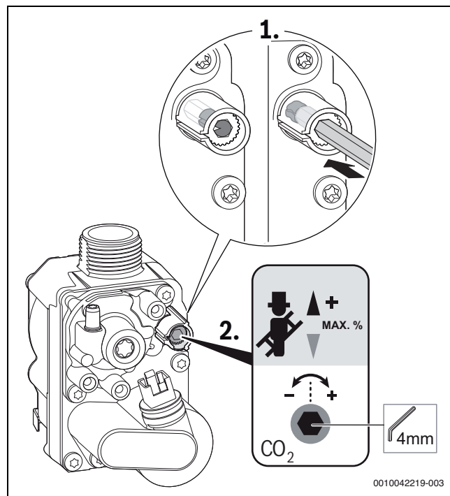
51. ábra A CO_2/O_2 -tartalom beállítása maximális névleges hőteljesítménynél, beállítható gázszerviz
