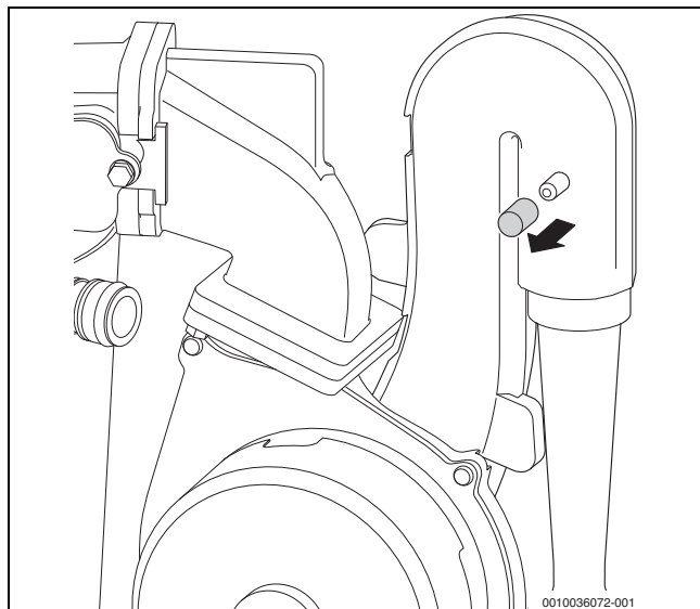
54. ábra Mérőcsok az előkeverőn
