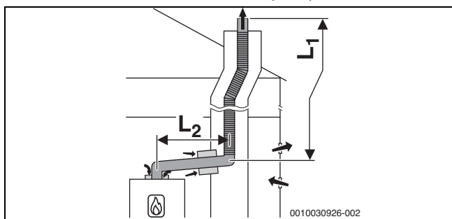
18. ábra B 23p /B 53p szerinti rugalmas füstgázvezetés kürtőben, nyílt égésterű levegőbevezetéssel a készüléken és koncentrikus összekötő darabbal a felállítási helyiség és a kürtő között
