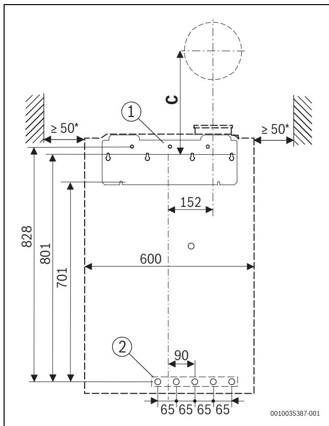
3. ábra Előlnézet, vízszintes hidraulikus csatlakozás(mm)
