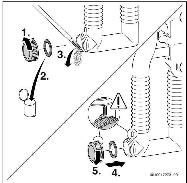
69. ábra A kondenzvíz szifon tisztítása
