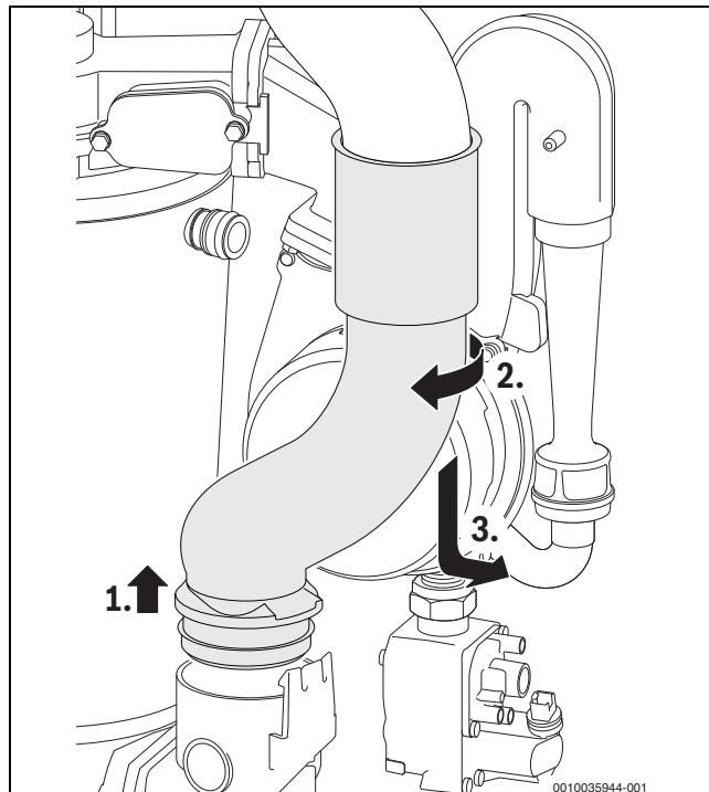
56. ábra A füstgázcső kiserelése
