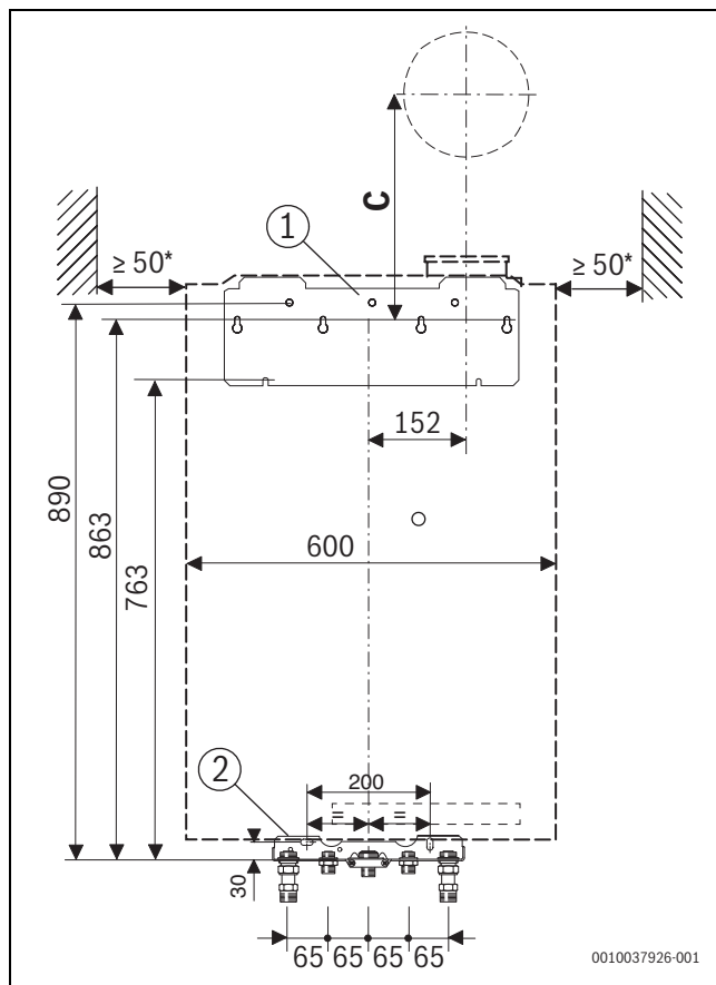
4. ábra Előlnézet, függőleges hidraulikus csatlakozás(mm)
