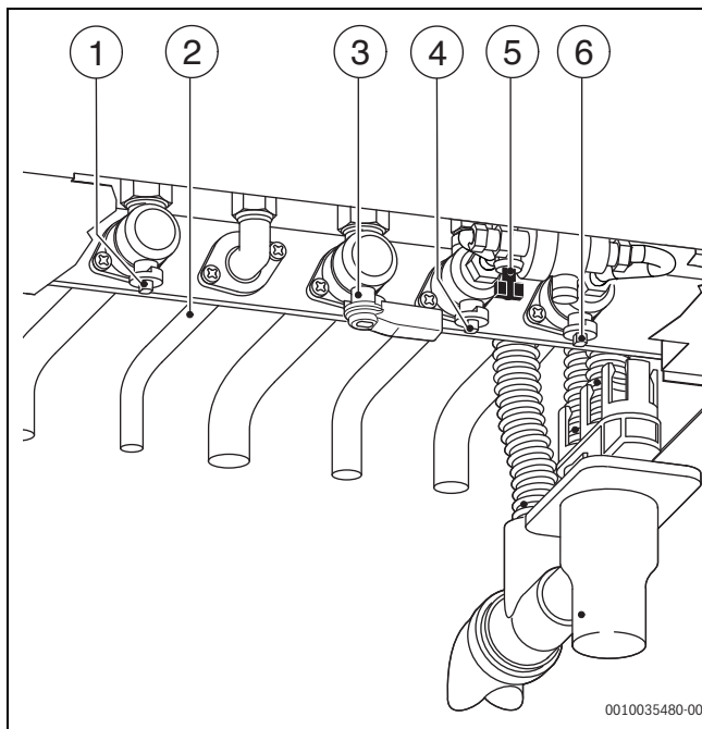
40. ábra Gáz- és vízdali csatlakozások
