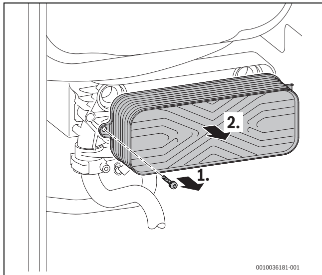
55. ábra A lemezes hőcserélő kiserelése
