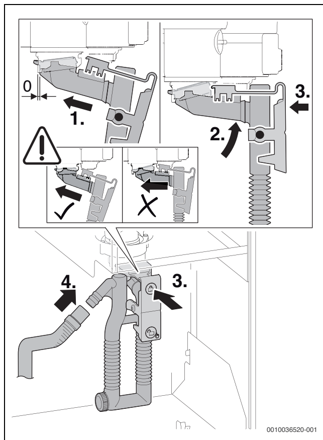
73. ábra A kondenzvízszfifon behelyezése
