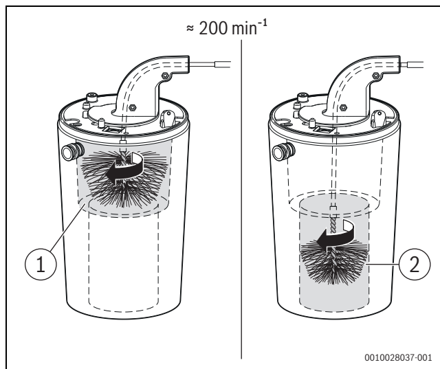
65. ábra A hőcserélő tisztítása (kb. 200 \text{ min}^{-1} , csak jobbra forgó)
