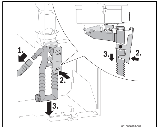
68. ábra A kondenzvíz szifon kiszérése
