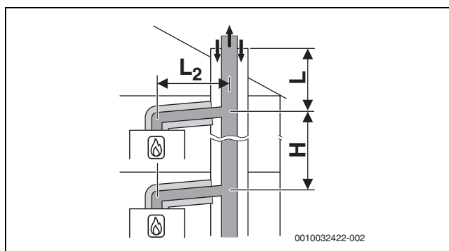
24. ábra Több fűtőkészülék bekötése a C (14)3x szerinti merev gyűjtő füstgázvezetéssel és koncentrikus levegő-/füstgázvezetéssel a felállítási helyiségben
