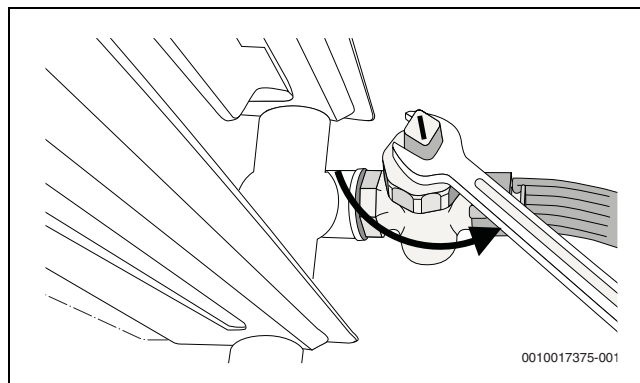
7. ábra A fűtési rendszer leürítése
