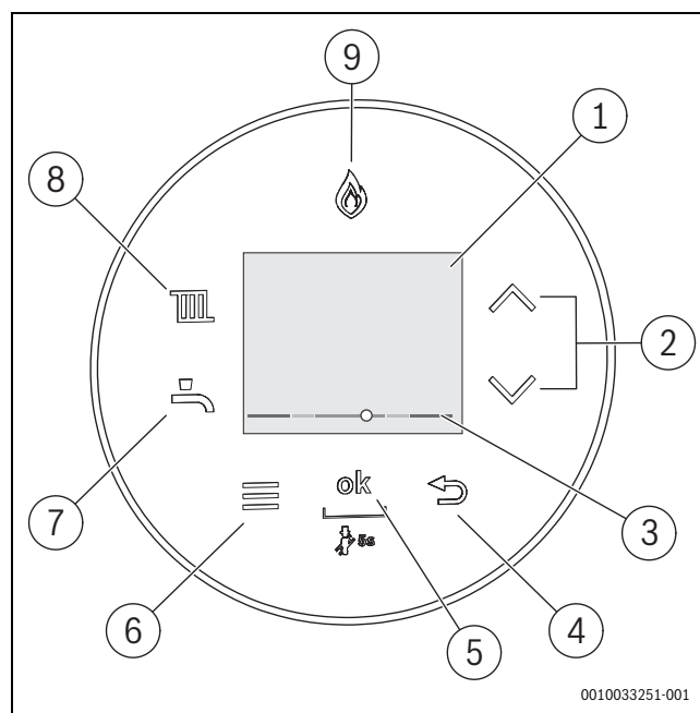
6. ábra Kezelőmező
