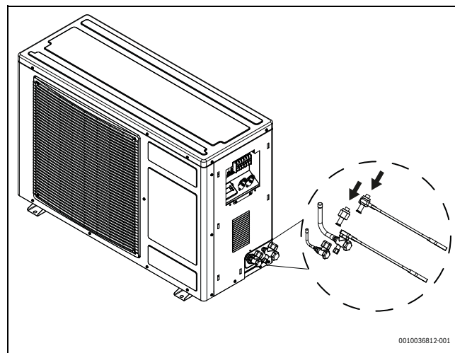
15. ábra Csavarozás
