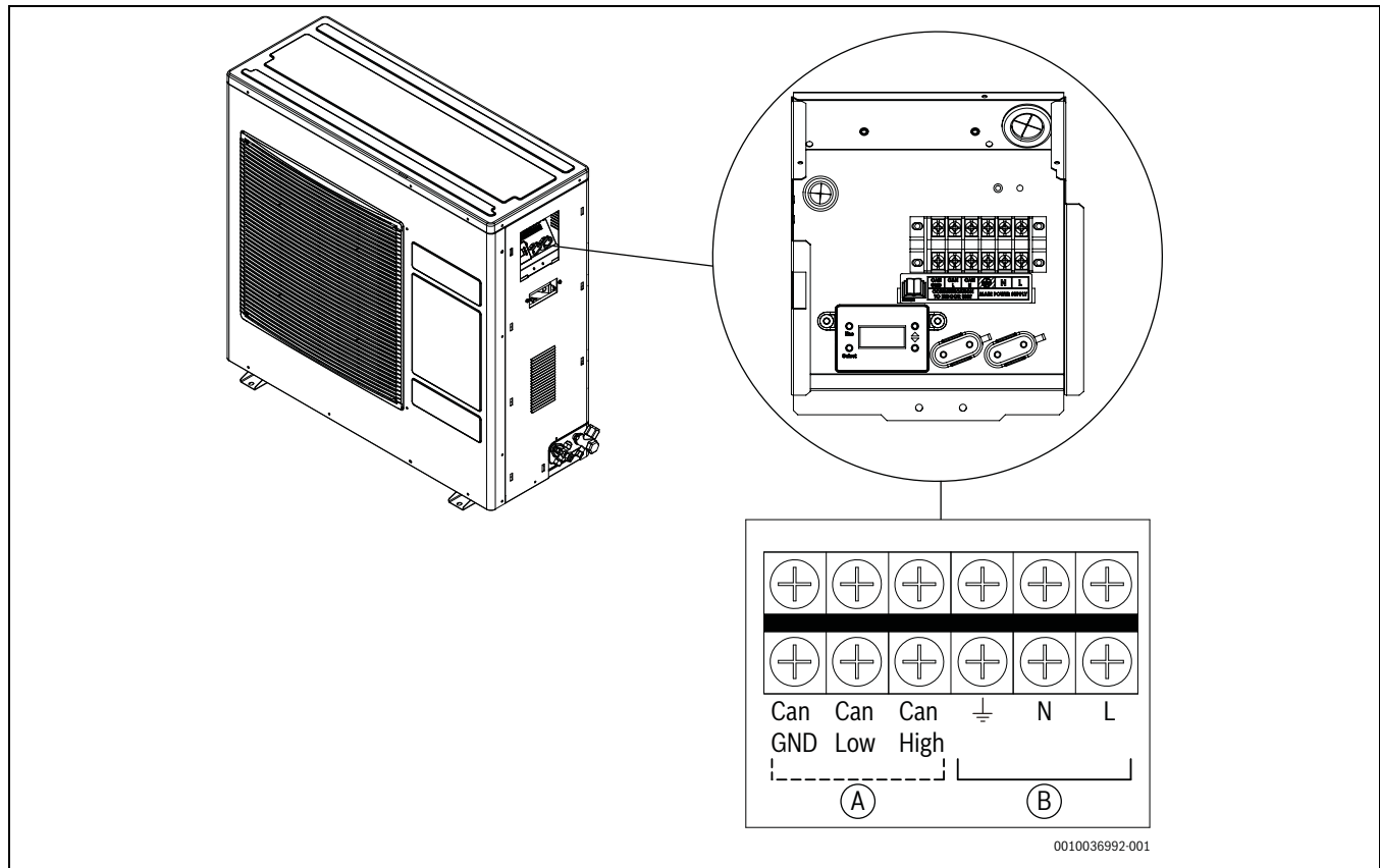
19. ábra Kábelcsatlakozások
