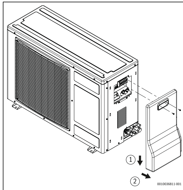
14. ábra Távolítsa el az oldalsó burkolatot
