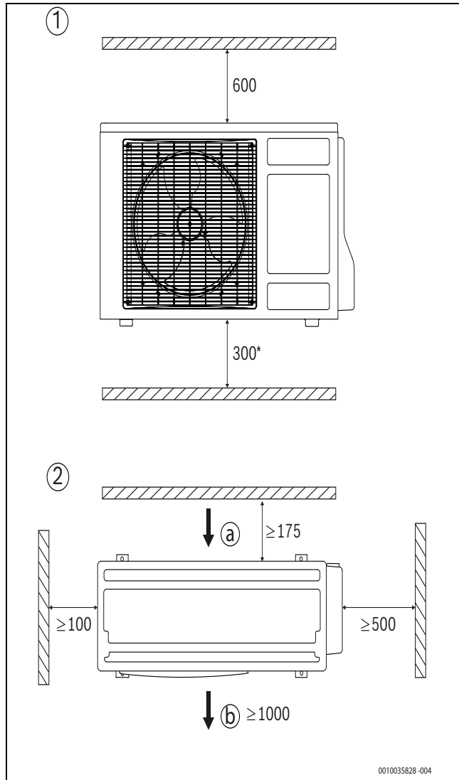
4. ábra Minimális távolságok (mm) 1)
