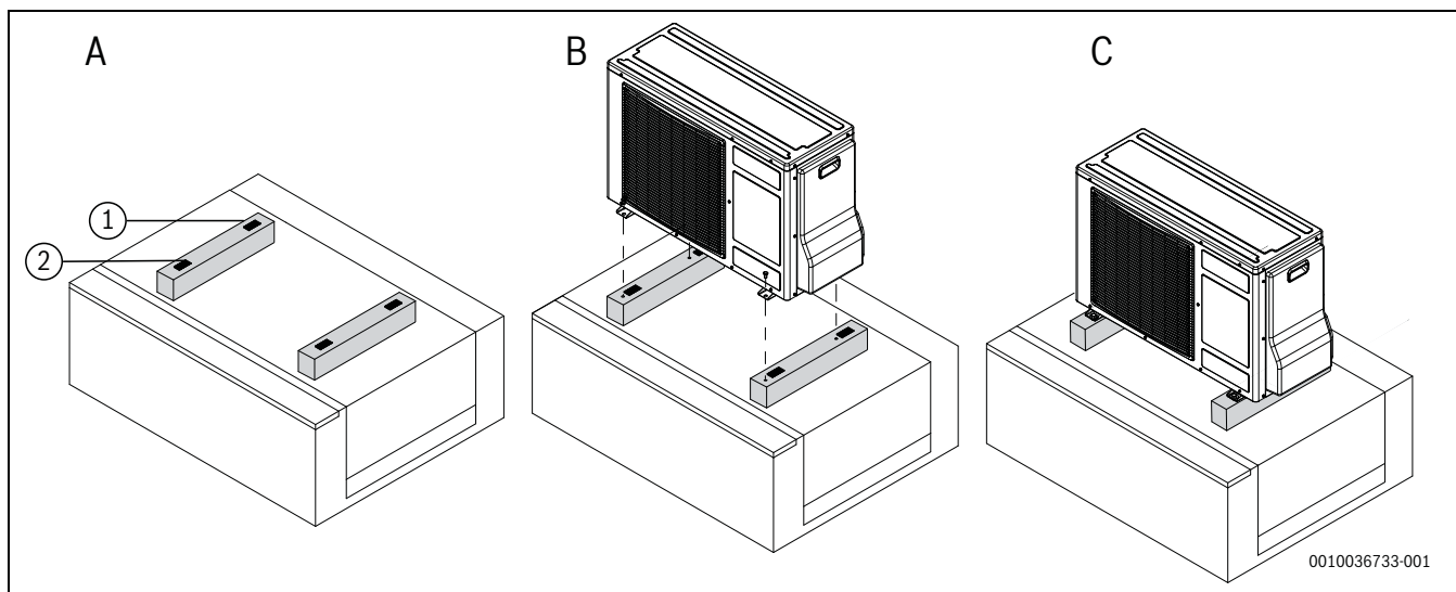
9. ábra Földön álló kültéri egység
