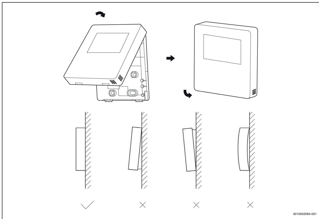
100. ábra A burkolatfedél felszerelése
