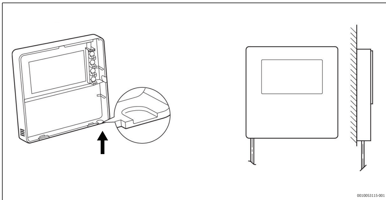
96. ábra A kábeldimenet pozicionálása
