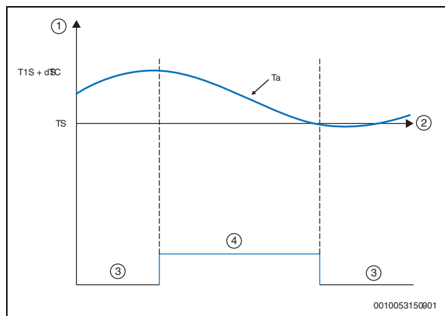
123. ábra Hűtési üzem – Levegő hőmérséklete (Ta)
