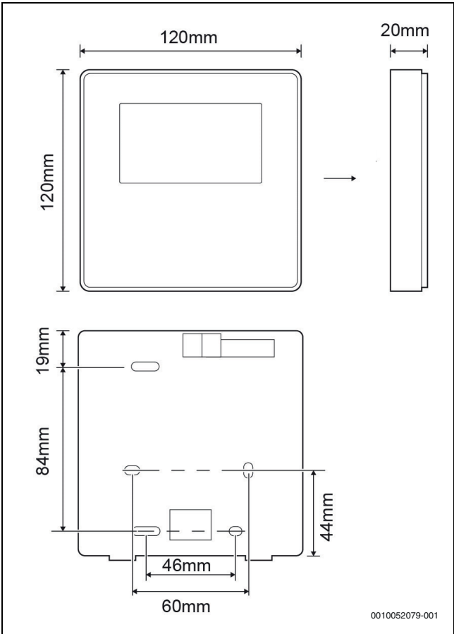
95. ábra A felhasználói felület beszerelése
