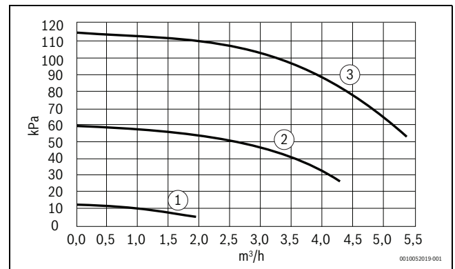
14. ábra CS2000AWF 18-30 R-T
