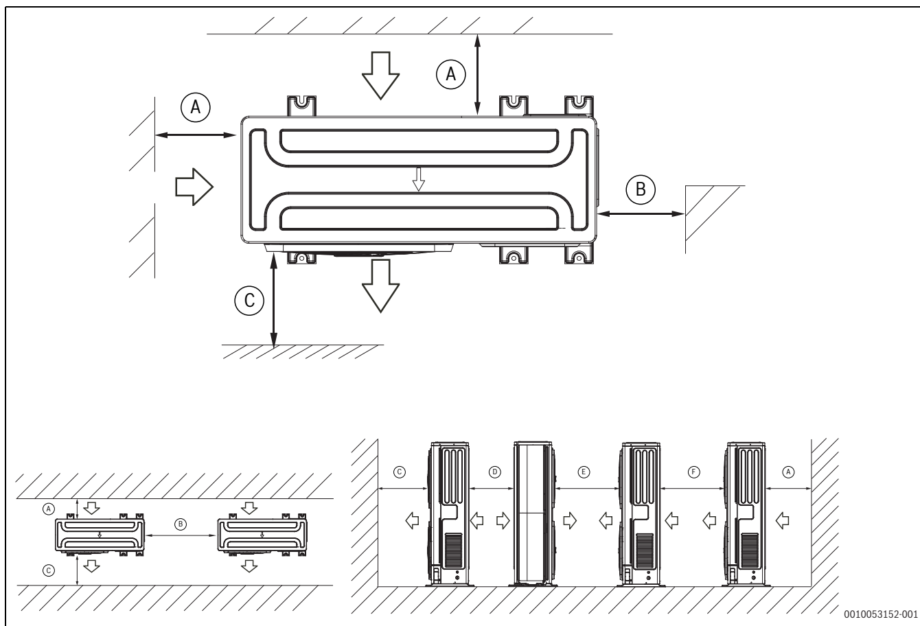
36. ábra Minimális távolságok
