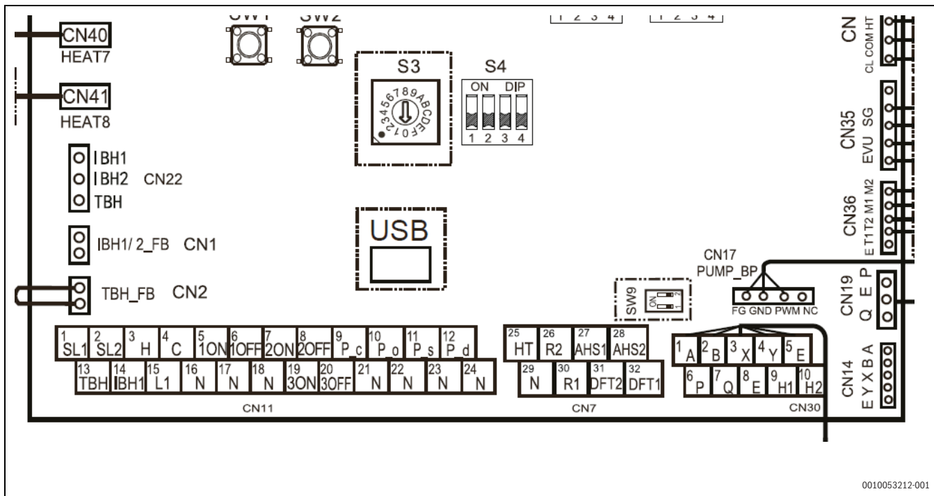
73. ábra Sorkapocsléc csatlakoztatása
