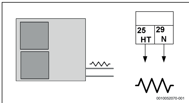
91. ábra Fagymentesítő fűtőberendezés csövekhez
