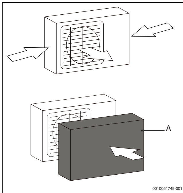
37. ábra Védje az egységet a különösen erős széltől.
