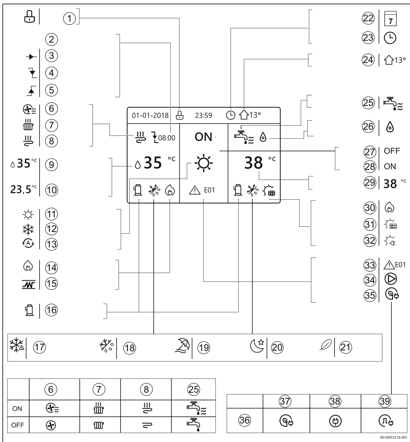
106. ábra Kijelző és ikonok
