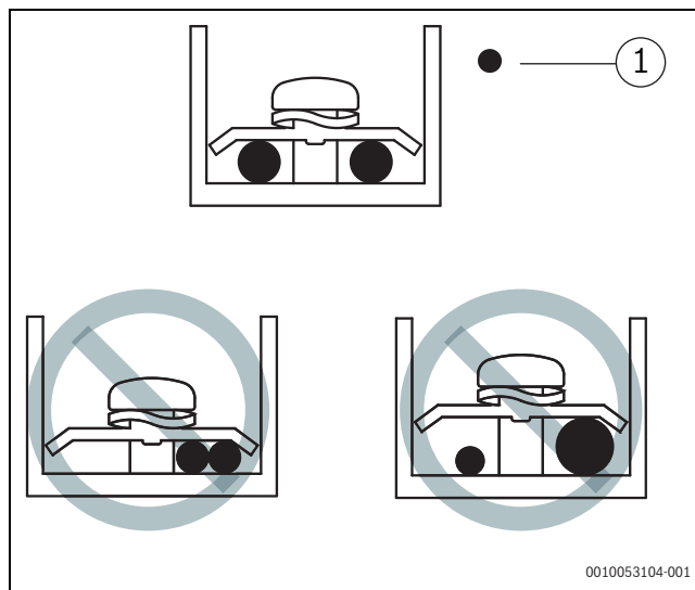
70. ábra Laza kábelezés esetén fennáll a túlmelegedés veszélye
