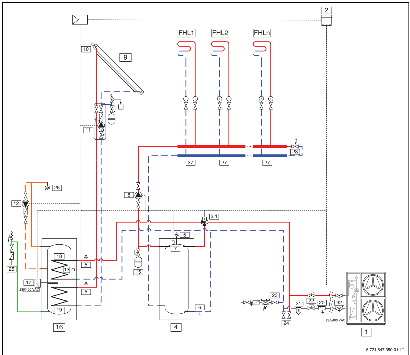
20. ábra Kültéri egység egy vagy több fűtőkörrel, melegvíz-tárolóval és napkollektorral (CS2000AWF 18-30 R-T)
