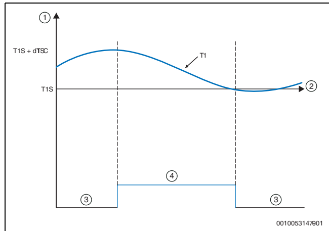
122. ábra Hűtési üzem – Előremenővíz- hőmérséklete (T1)
