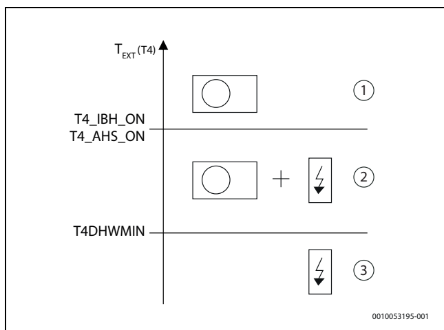
134. ábra Nagyon alacsony külső hőmérséklet
