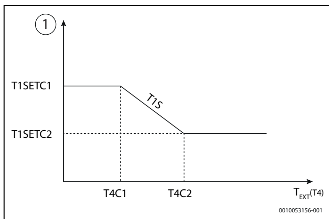
124. ábra Hűtési üzem – Az elosztórendszer beállítása
