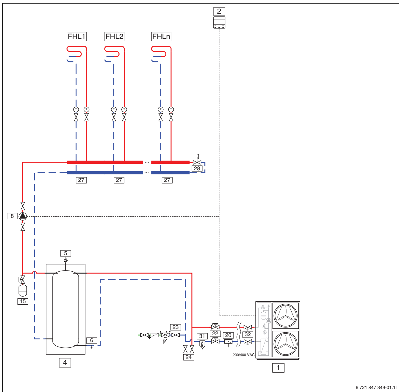
19. ábra Kültéri egység egy vagy több fűtőkörrel (CS2000AWF 18 -30 R-T)
