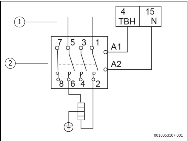
75. ábra 2. TÍPUSÚ vezérlőjel
