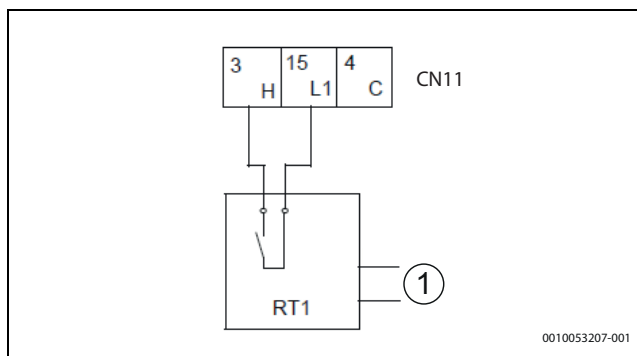
102. ábra Zóna termosztát – B módszer
