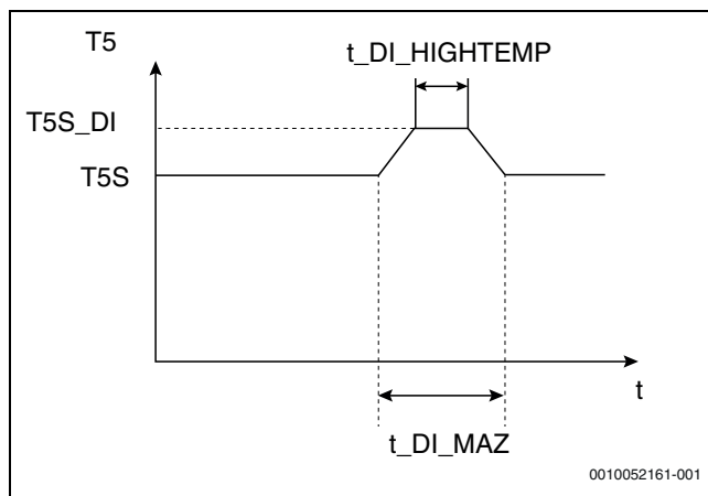
119. ábra 1.15 t_DI_MAGHŐM
