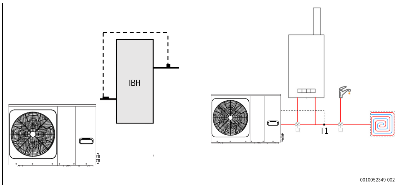
133. ábra A kiegészítő hőforrás beállításai
