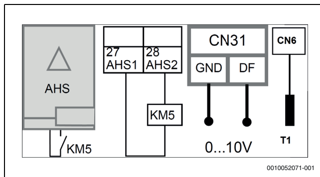
92. ábra Kiegészítő kazán
