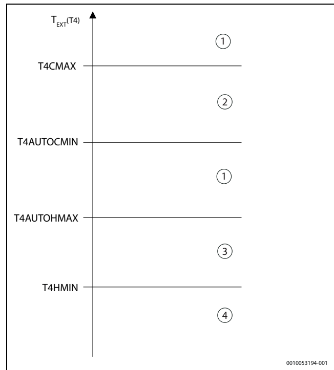
128. ábra AUTO üzemi működés
