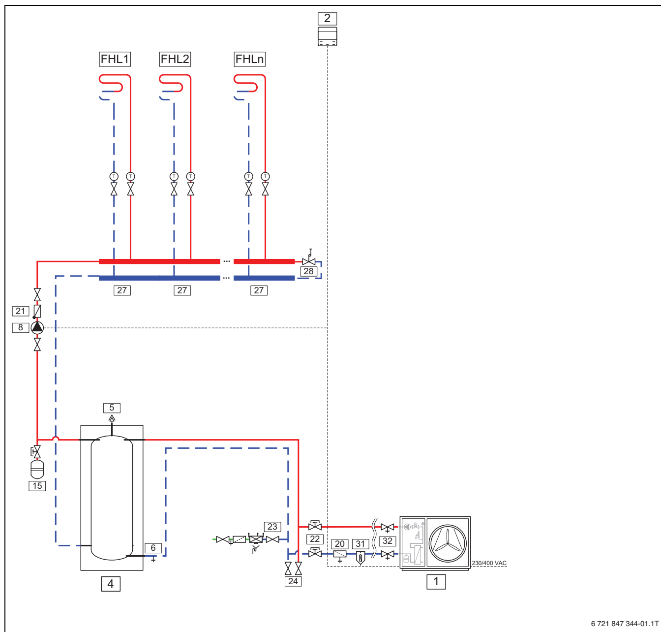
16. ábra Kültéri egység egy vagy több fűtőkörrel (CS2000AWF 4-6 R-S, CS2000AWF 8-10 R-S, CS2000AWF 12-16 R-S/T)
