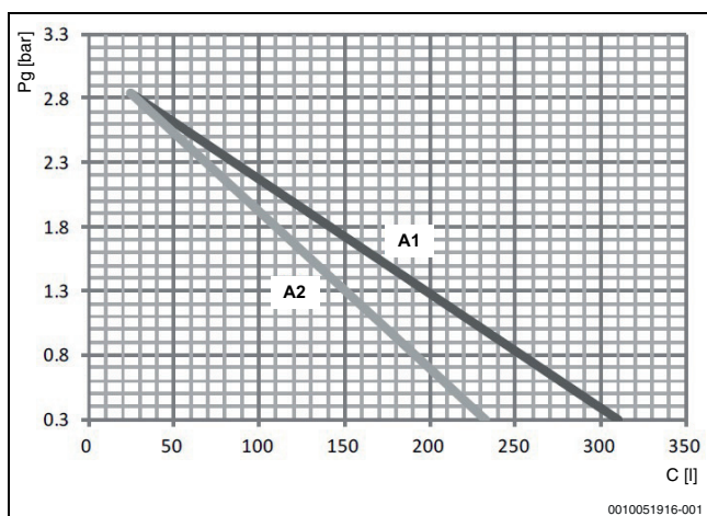
57. ábra Maximális vízirtalom
