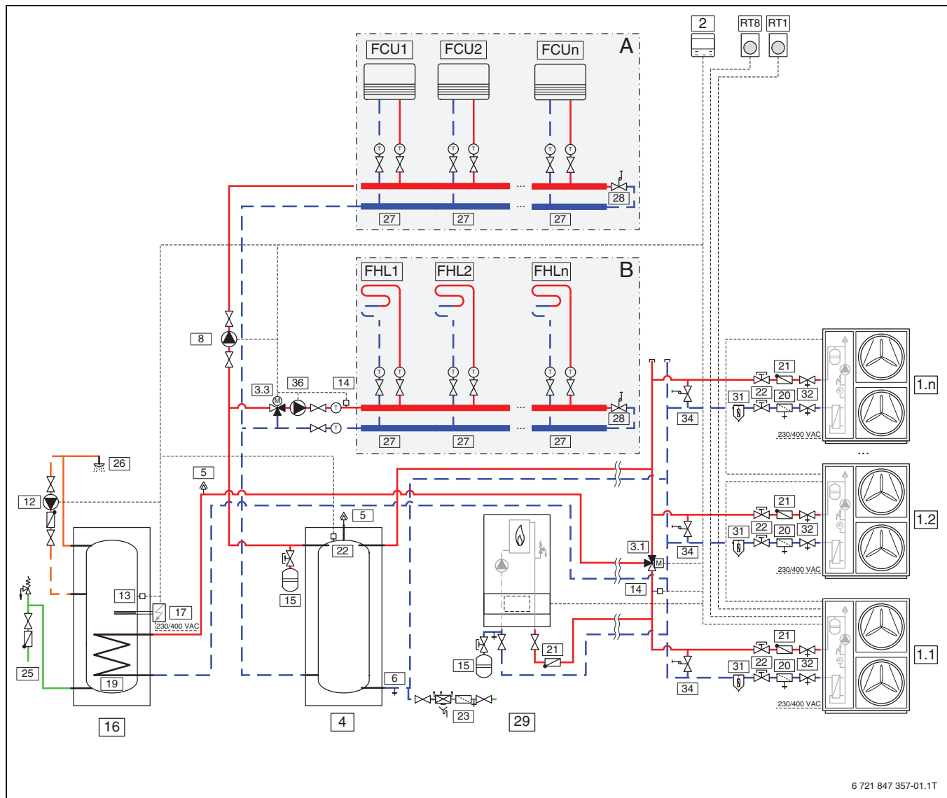
27. ábra Kültéri egység egy vagy több fűtőkörrel, külső kiegészítő fűtőberendezéssel, melegvíz-tárolóval és kaszkárendszerrel (CS2000AWF 18-30 R-T)
