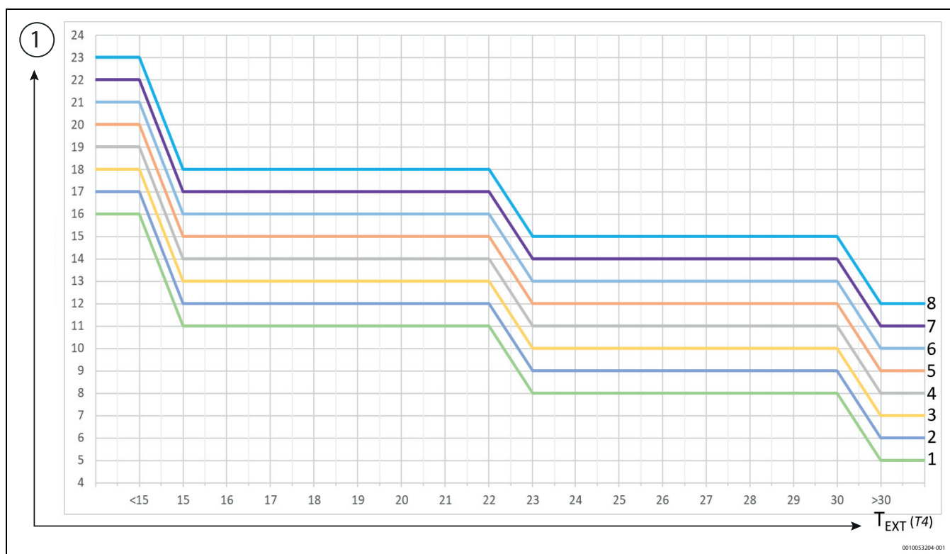
149. ábra Hűtési üzem végponti elosztással rendelkező rendszerekben
