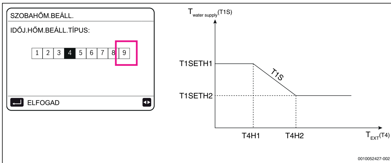
147. ábra Testre szabható görbe – külső levegő hőmérséklete ( T4H1 , T4H2 ) és vízhozzávetés ( T1SETH1 , T1SETH2 )
