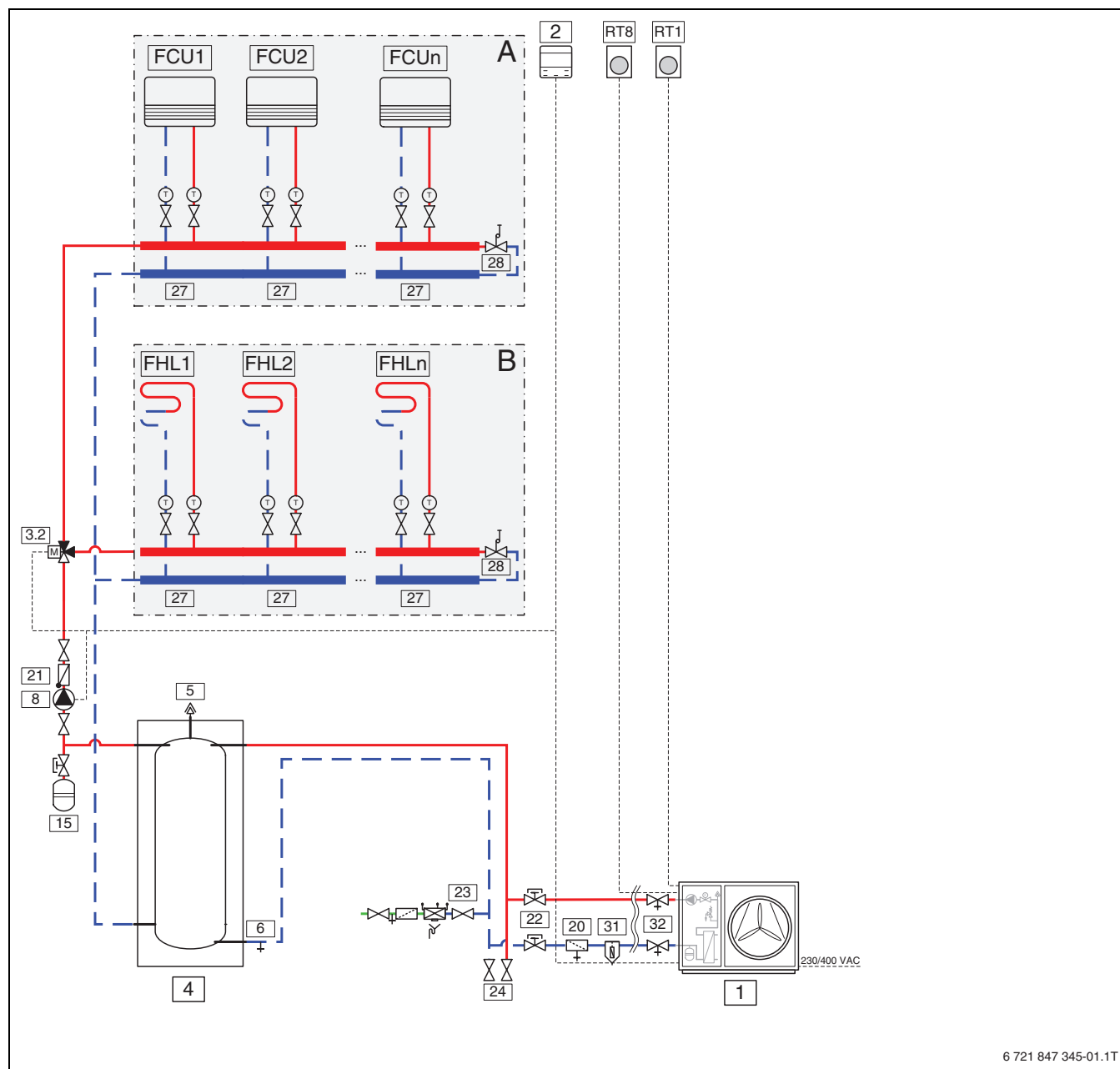
17. ábra Kültéri egység egy vagy több fűtőkörrel, padlófűtéssel és fan-coil egységgel (CS2000AWF 4-6 R-S, CS2000AWF 8-10 R-S, CS2000AWF 12-16 R-S/T)
