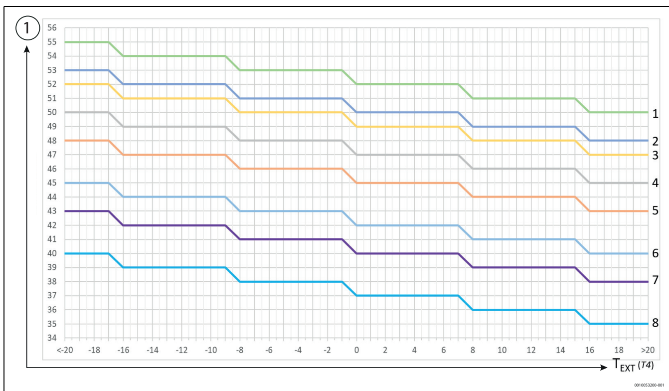
146. ábra Fűtési üzem végponti elosztással rendelkező rendszerekben
