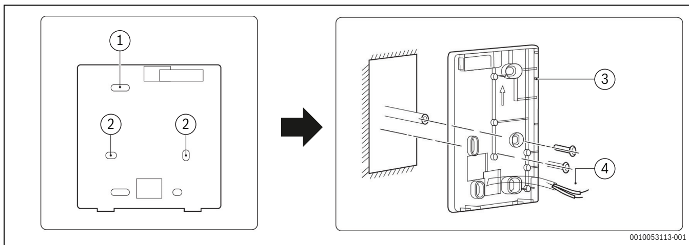
98. ábra Beszerelés a 86 kapcsolószekrénybe
