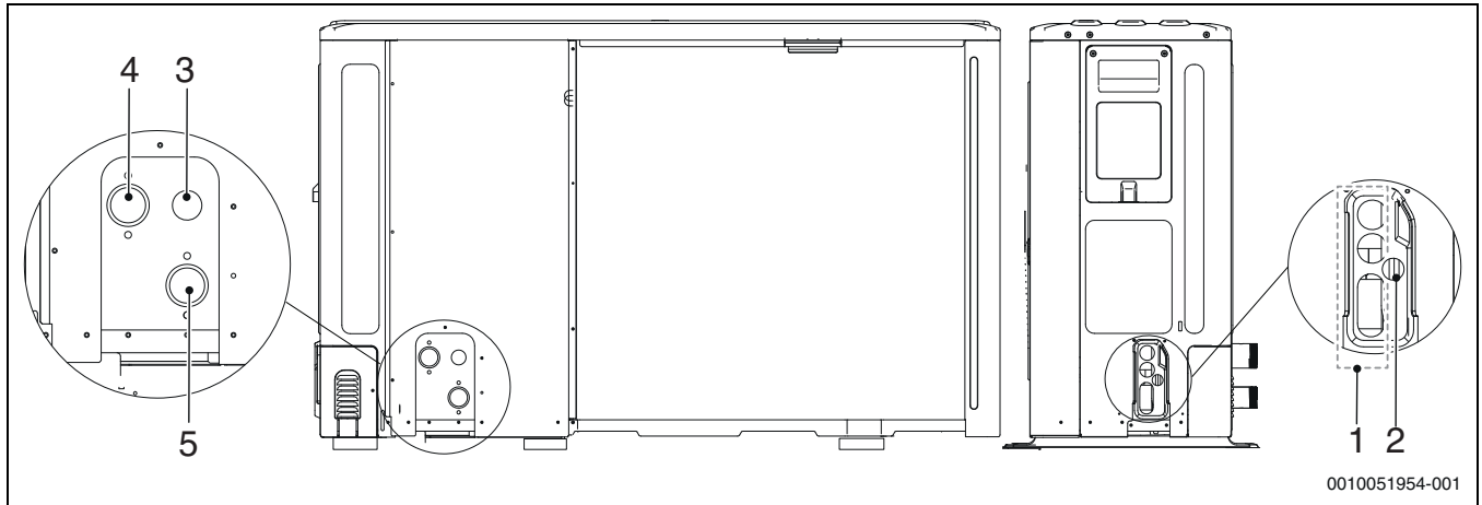
65. ábra CS2000AWF 8 R-S és CS2000AWF 16 R-S/CS2000AWF 16 R-T közötti méretek
