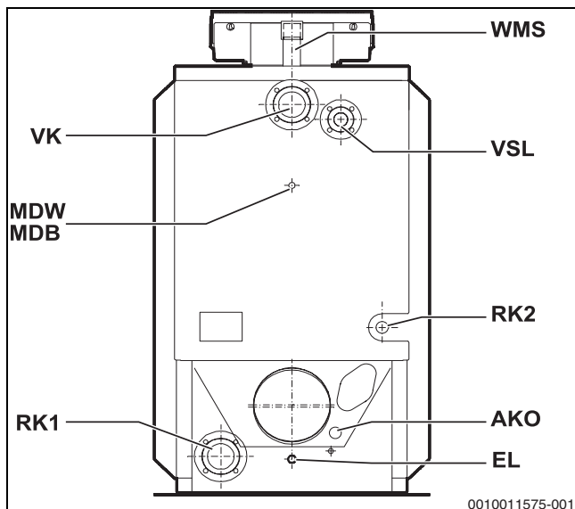
12. ábra Kazán csatlakozások
