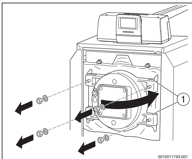
26. ábra Tüztérajtó nyitása
