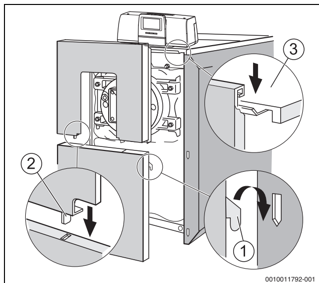
25. ábra Az alsó és a felső homlokfal rögzítése
