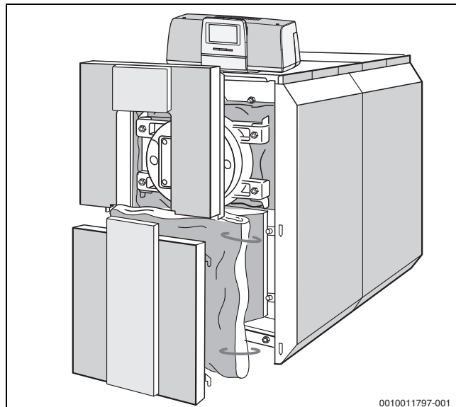
44. ábra A homlokfal és az előlő hőszigetelés leemelése
