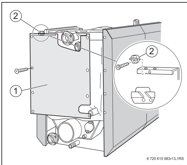
21. ábra A hátfal felcsavarozása (400 kW és 640 kW közötti kazánméret)
