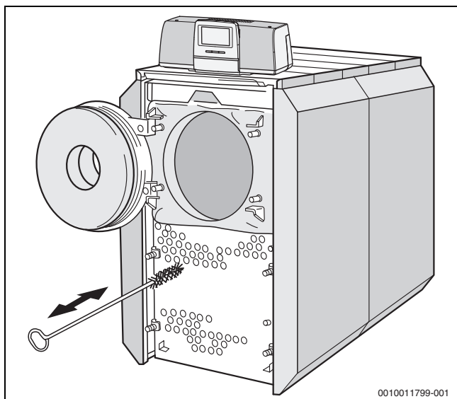
46. ábra Kazán tisztítása tisztítókefével
