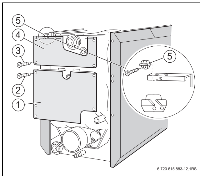
20. ábra A 2-részes hátfal felcsavarozása (145 kW és 310 kW közötti kazánméret)
