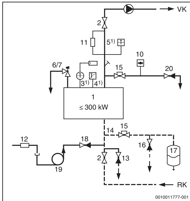
49. ábra Biztonságtechnikai felszerelés az EN 12828:2012 szerint ≤ 300 kW kazánokhoz, ≤ 110 °C biztonsági hőmérséklet-határolóval (STB)
