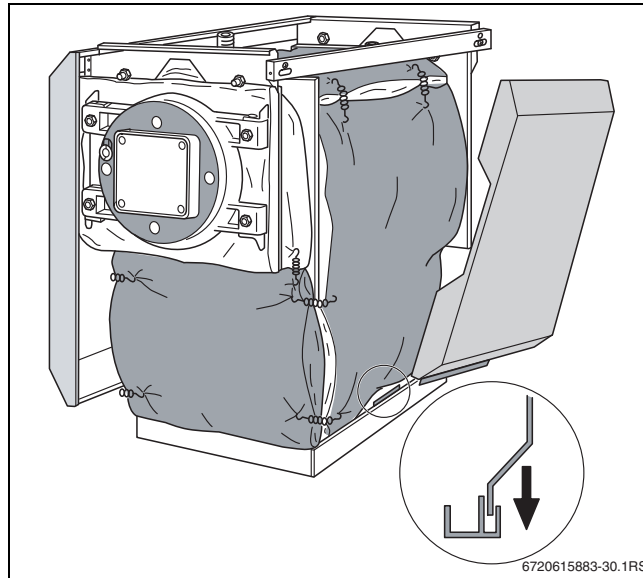
18. ábra Az oldalfalak behelyezése
