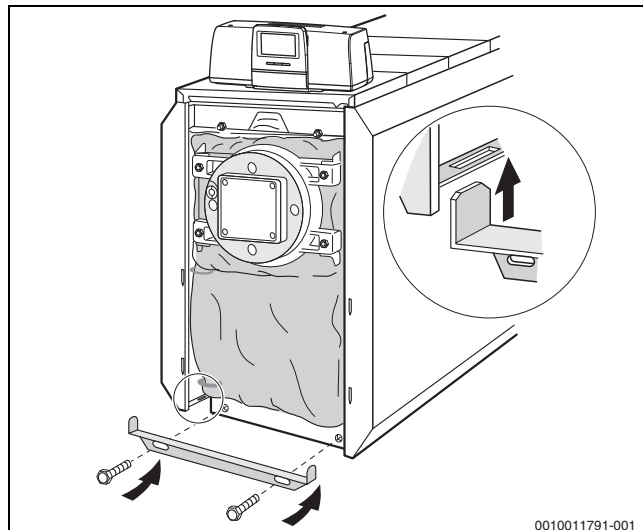
24. ábra Az alsó kereszttartó rögzítése csavarokkal
