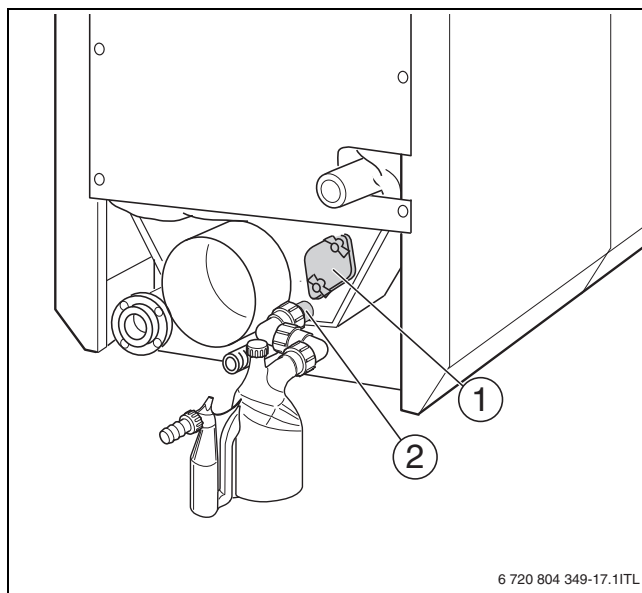
47. ábra Füstgázgyűjtő tisztítófedél
