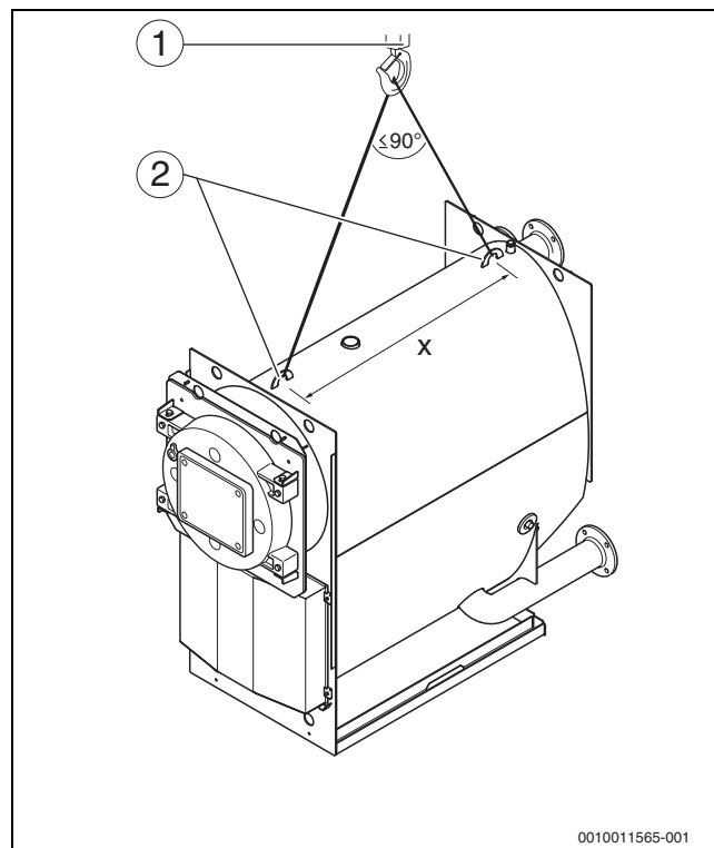
4. ábra Emelje meg a kazánt a daruval
