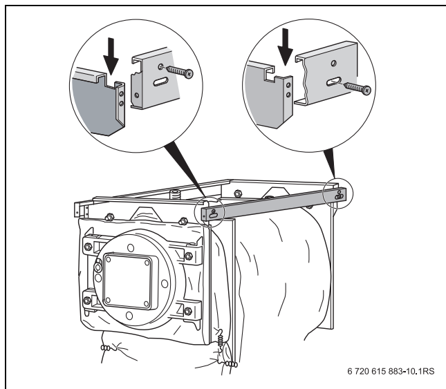
17. ábra Az oldalsó kereszttartók beakasztása és összecsavarozása
