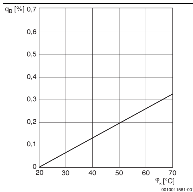
52. ábra Az üzemkészség elvesztése a közepes kazánvíz hőmérséklettől függően
