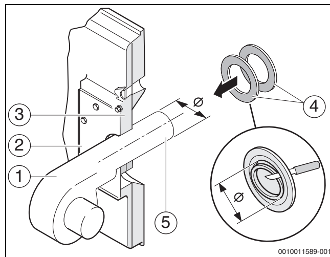
28. ábra Az égő felszerelése
