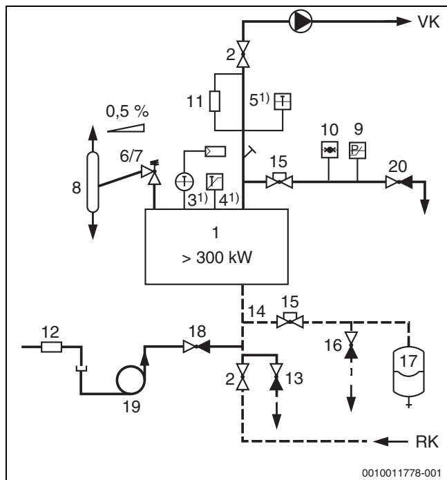
50. ábra Biztonságtechnikai felszerelés az EN 12828:2012 szerint > 300 kW kazánokhoz, ≤ 110 °C biztonsági hőmérséklet-határolóval (STB)
