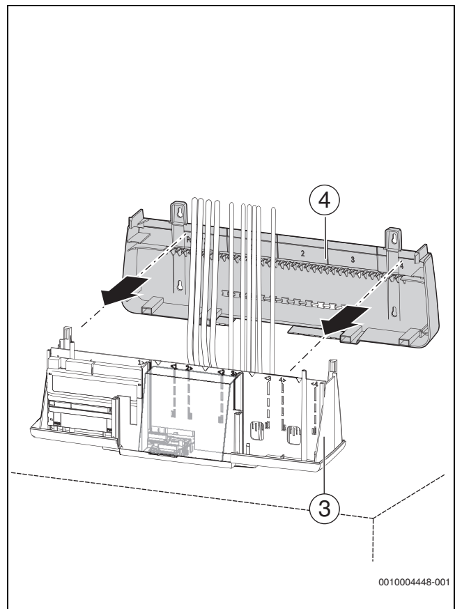
38. ábra Szerelés a kazánra, hátfal rögzítése
