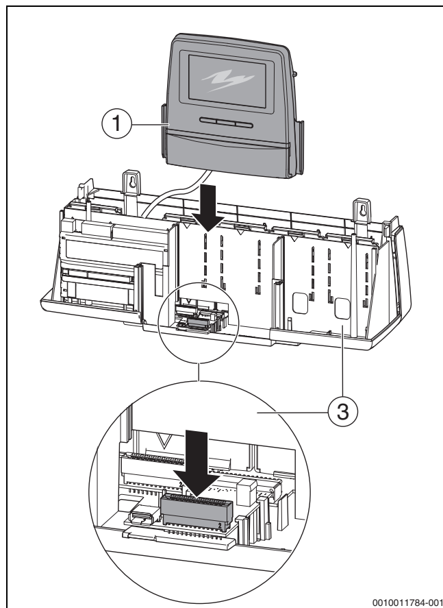
42. ábra A vezérlőelektronika bedugása a ház alsó részénél
