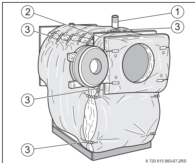
10. ábra A hőszigetelő felhelyezése és rögzítése
