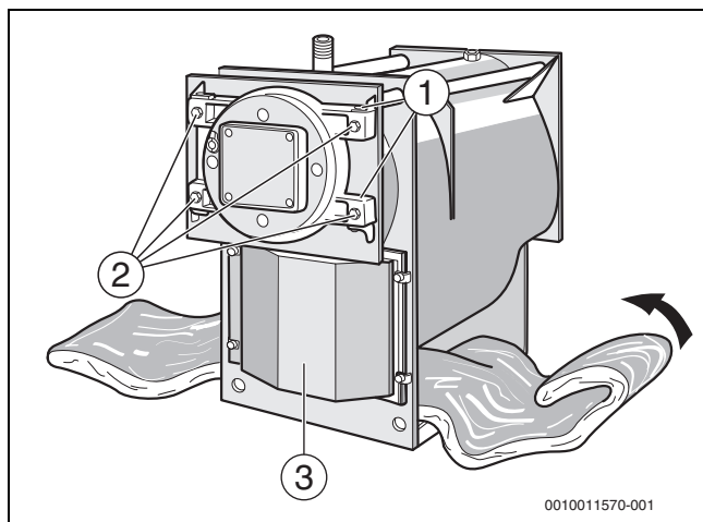
9. ábra A hőszigetelő borítás áttolása a kazán alatt
