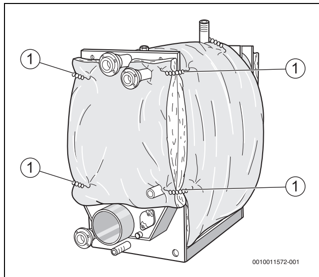
11. ábra A hátfal hőszigetelőjének felhelyezése és rögzítése
