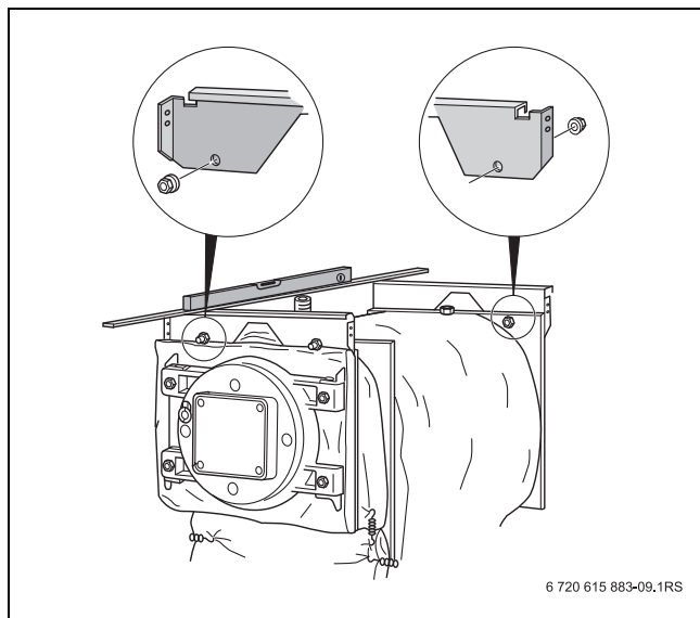
16. ábra Az elülső és a hátsó kereszttartó behelyezése és összecsavarozása
