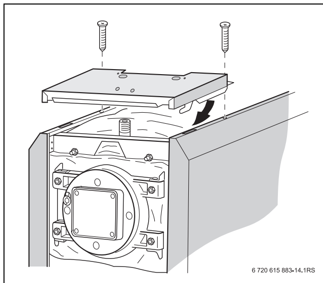
23. ábra A kazán elülső tetőburkolatának felszerelése
