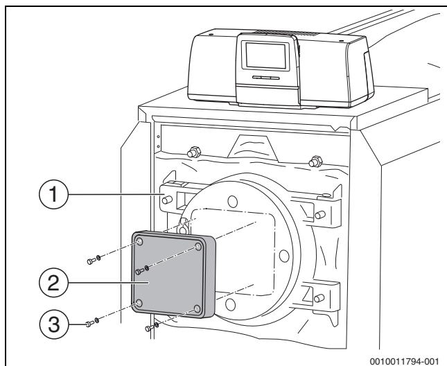
27. ábra Az égőlap felszerelése
