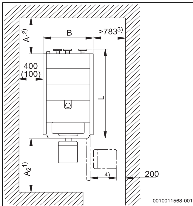
7. ábra Felállítási helyiség méretei mm-ben (→ 10. tábl., 16. oldal)
