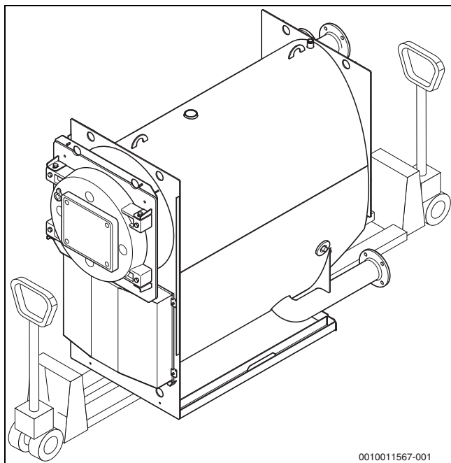
6. ábra Kazán szállítása két emelőkocsival
