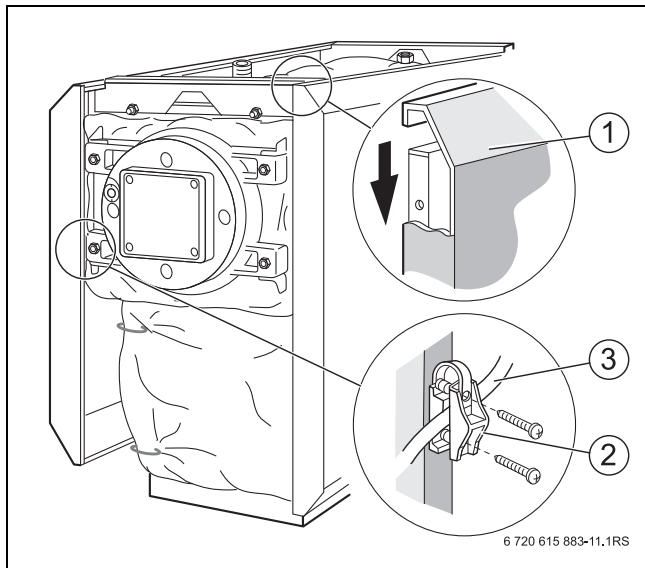
19. ábra Az oldalfalak beakasztása és az égőkábel elhelyezése
