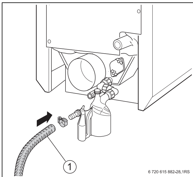
14. ábra A semlegesítő berendezés beszerelése
