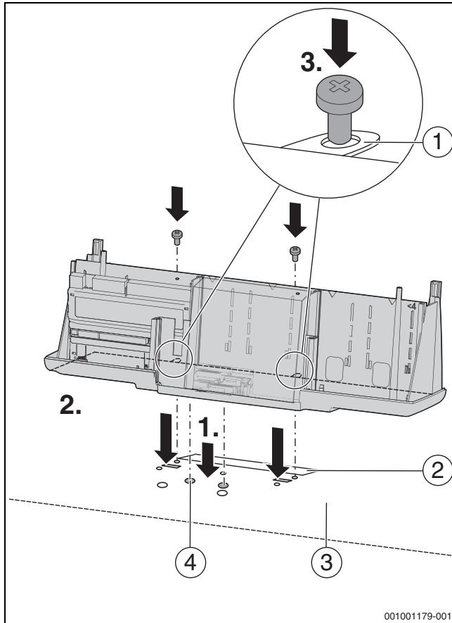
36. ábra A vezérlőelektronika felszerelése
