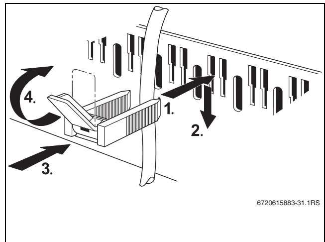
37. ábra Biztosítsa a kábelt a kábelbilincssel
