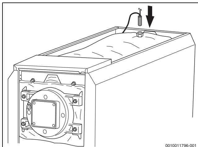
30. ábra Hőmérséklet-érzékelő bevezetése a merülőhüvelybe
