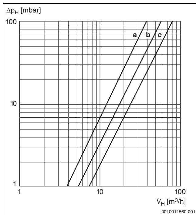
51. ábra Vízoldali átfolyási ellenállás
