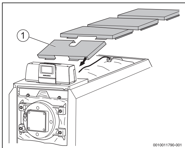
22. ábra Tetőburkolatok felhelyezése - elvi ábrázolás
