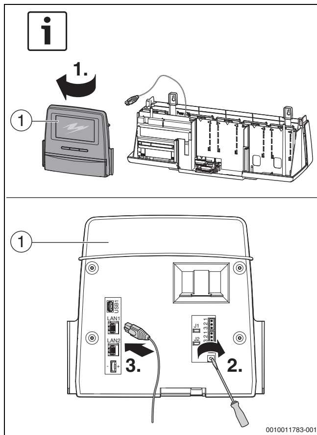
41. ábra Vezérlőelektronika címének beállítása
