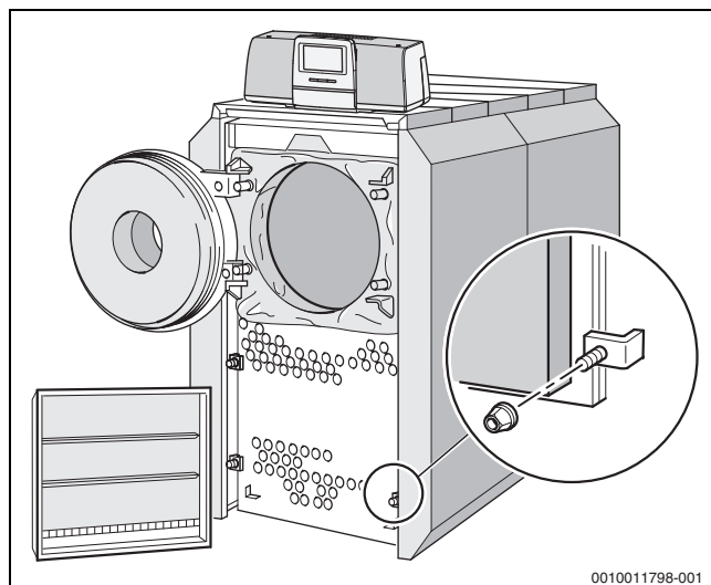
45. ábra A terelőburkolat levétele és a tüztérajtó kinyitása
