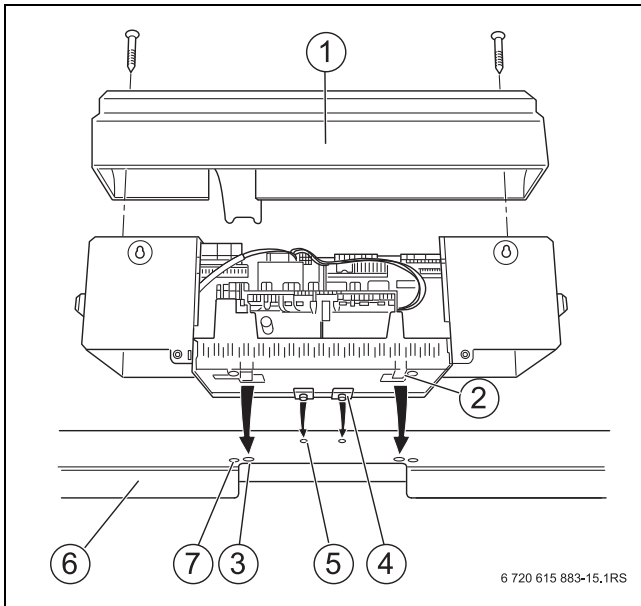
32. ábra A vezérlőelektronika felszerelése
