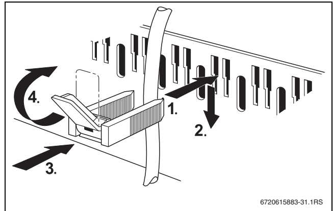
34. ábra Biztosítsa a kábelt a kábelbilincssel
