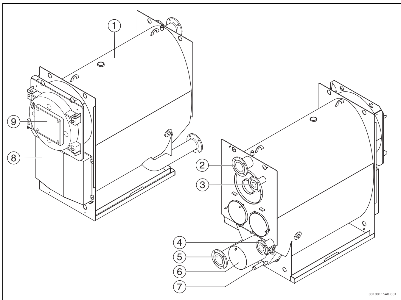
2. ábra Kazán áttekintése
