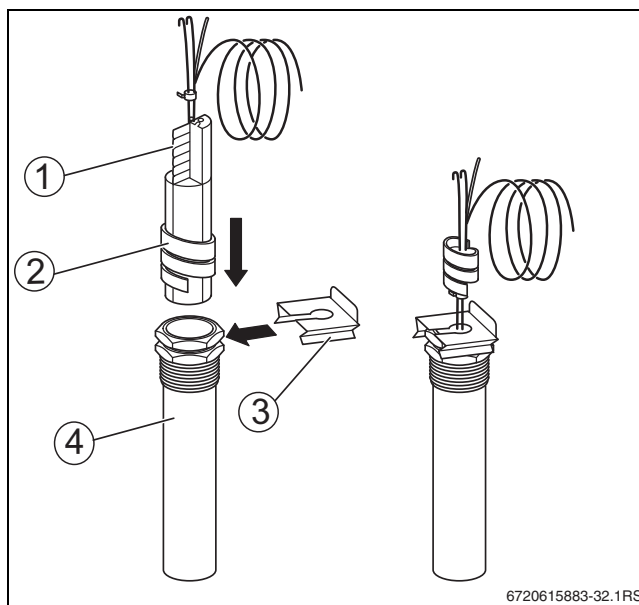
31. ábra A műanyag spirál behelyezése a merülőhüvelybe
